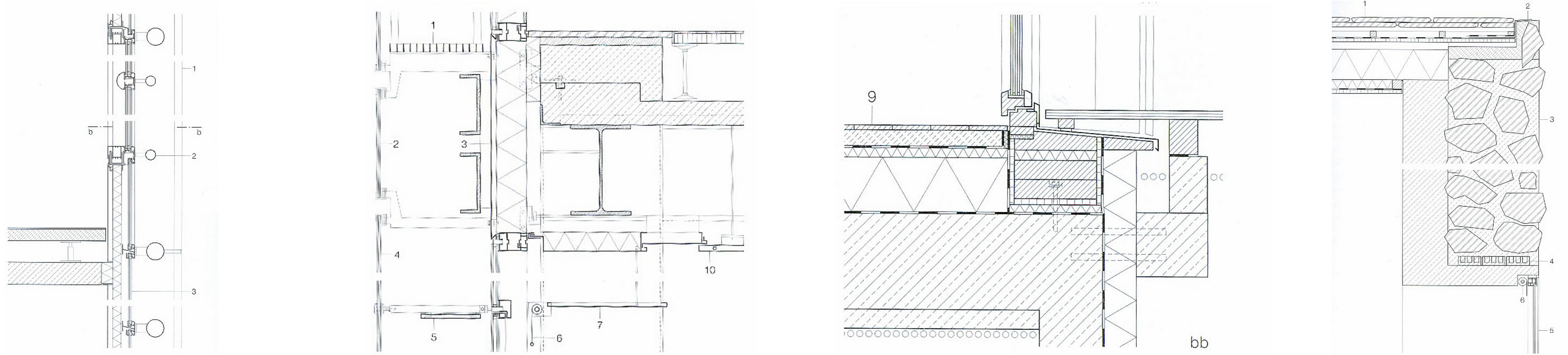
Zeichenstil - Beispiele aus Fachzeitschrift "Detail" (2007)
